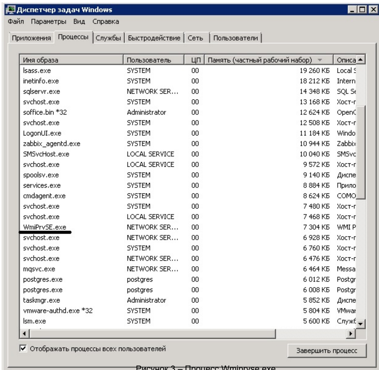
Рисунок 3 – Процесс WmiPrvse.exe
