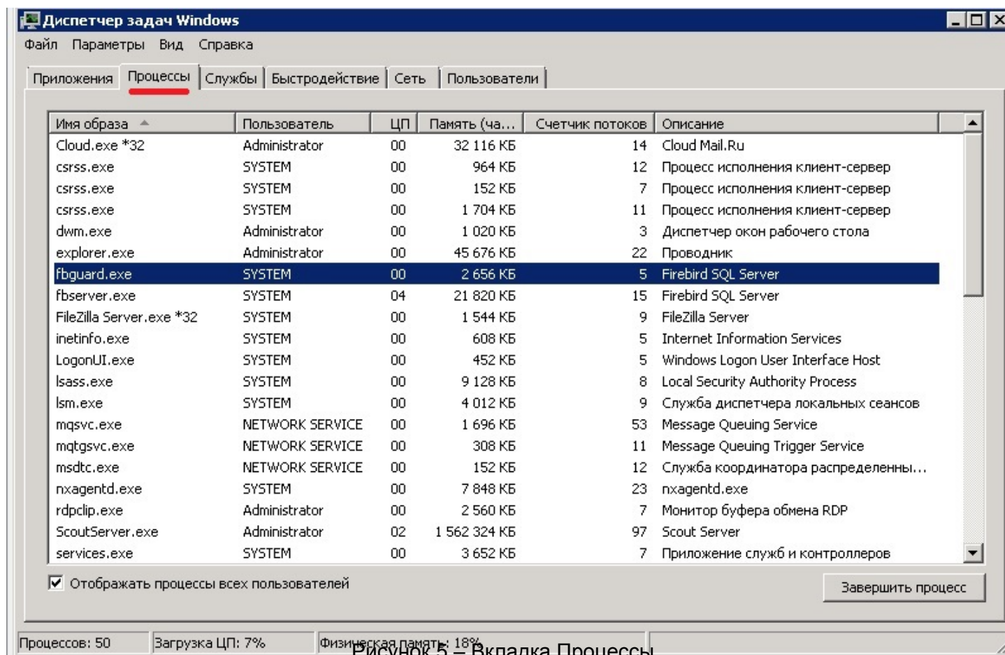
Рисунок 5 – Вкладка Процессы
