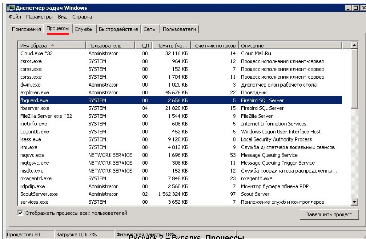
Рисунок 2 – Вкладка Процессы
